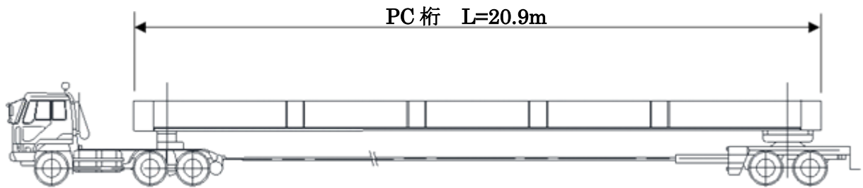
PC桁 運搬荷姿図
